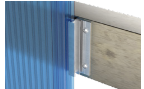
Förlängt fästbeslag.
