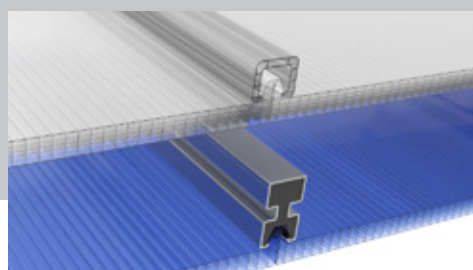
Fästbeslag 4328.
